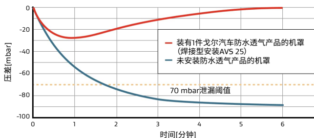
温度骤变所致的压差
