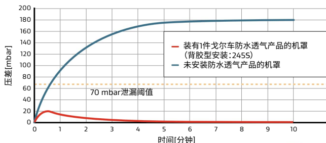
发热所导致的压差
