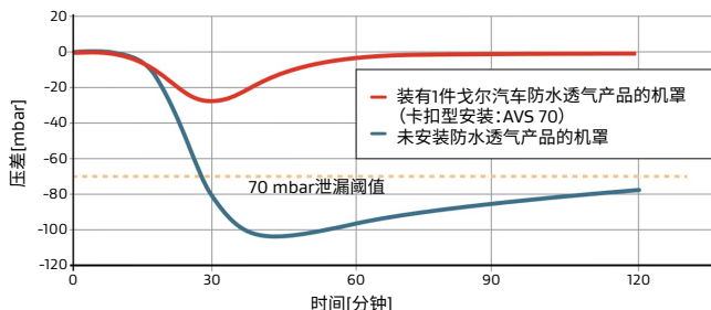
海拔高度和温度变化所致的压差
