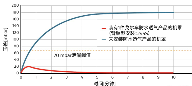
发热所导致的压差
