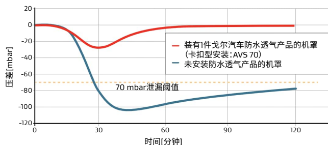
海拔高度和温度变化所致的压差
