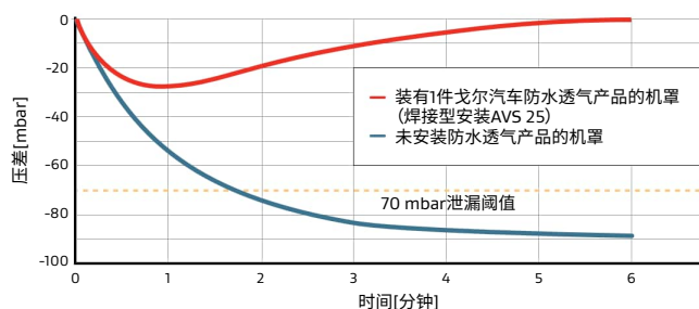
温度骤变所致的压差
